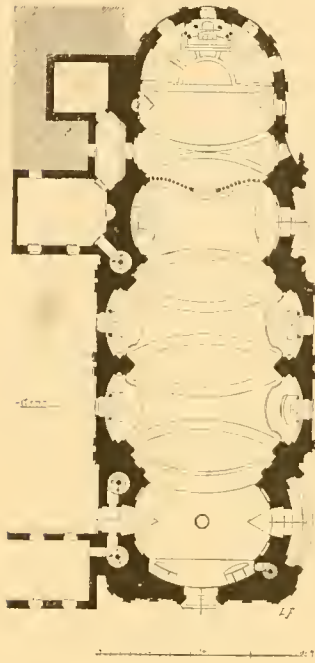
Fig. 57. St. Margareth in Břevnov. Grundriß.
